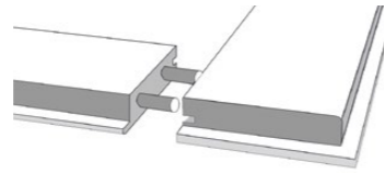
RAHMENAUFBAU Aufbauelemente, die durch Montagebolzen verbunden sind
