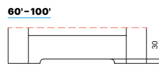
HÖHE DES LÜFTUNGSUNTERSCHNITTS BEI RAHMENTÜREN, FÜR BREITEN 60'-100' 2
