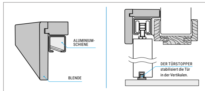
VERTIKALER QUERSCHNITT DES SCHIEBESYSTEMS
